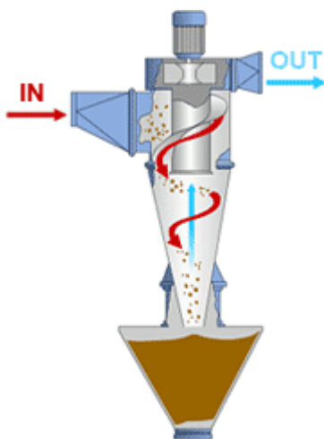
Слика 15 Циклонски собирач на прашина
