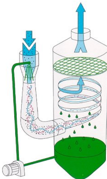
Слика 19 Вентури скруббер
