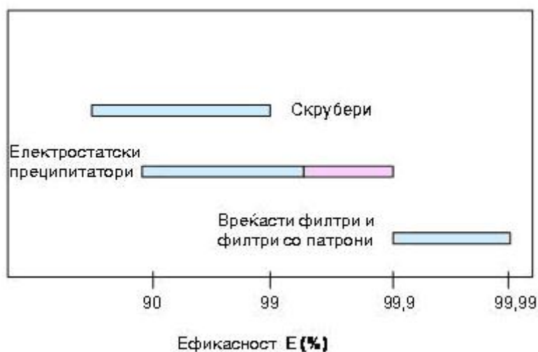
Слика 23 Вообичаен опсег на ефикасност на најчесто применуваната опрема за намалување на цврсти честички
