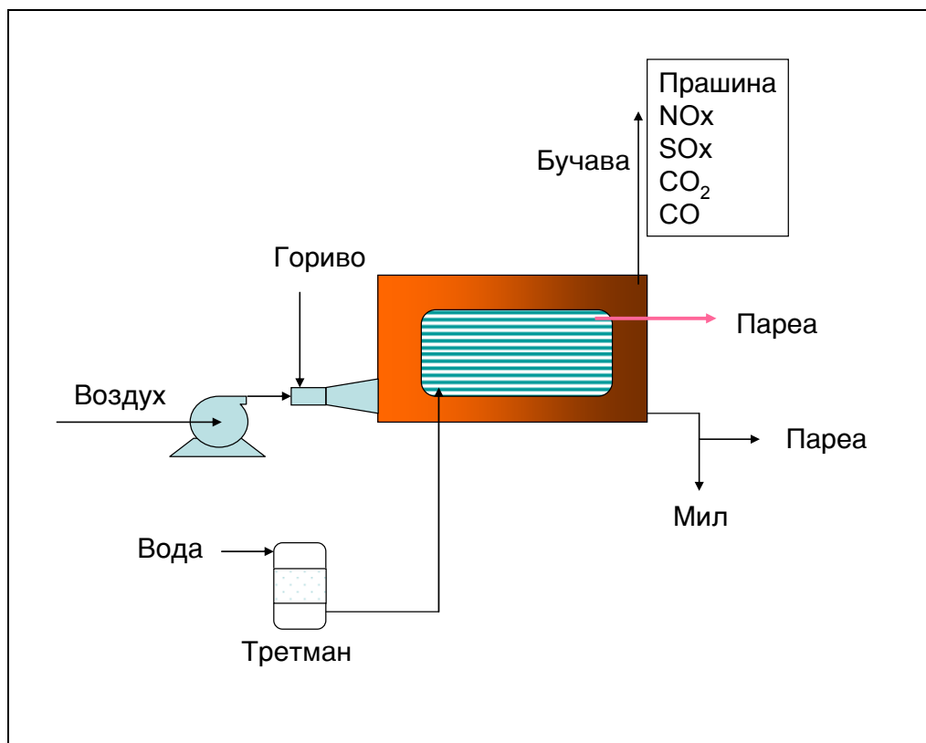
Слика 2 Единична операција - котел
