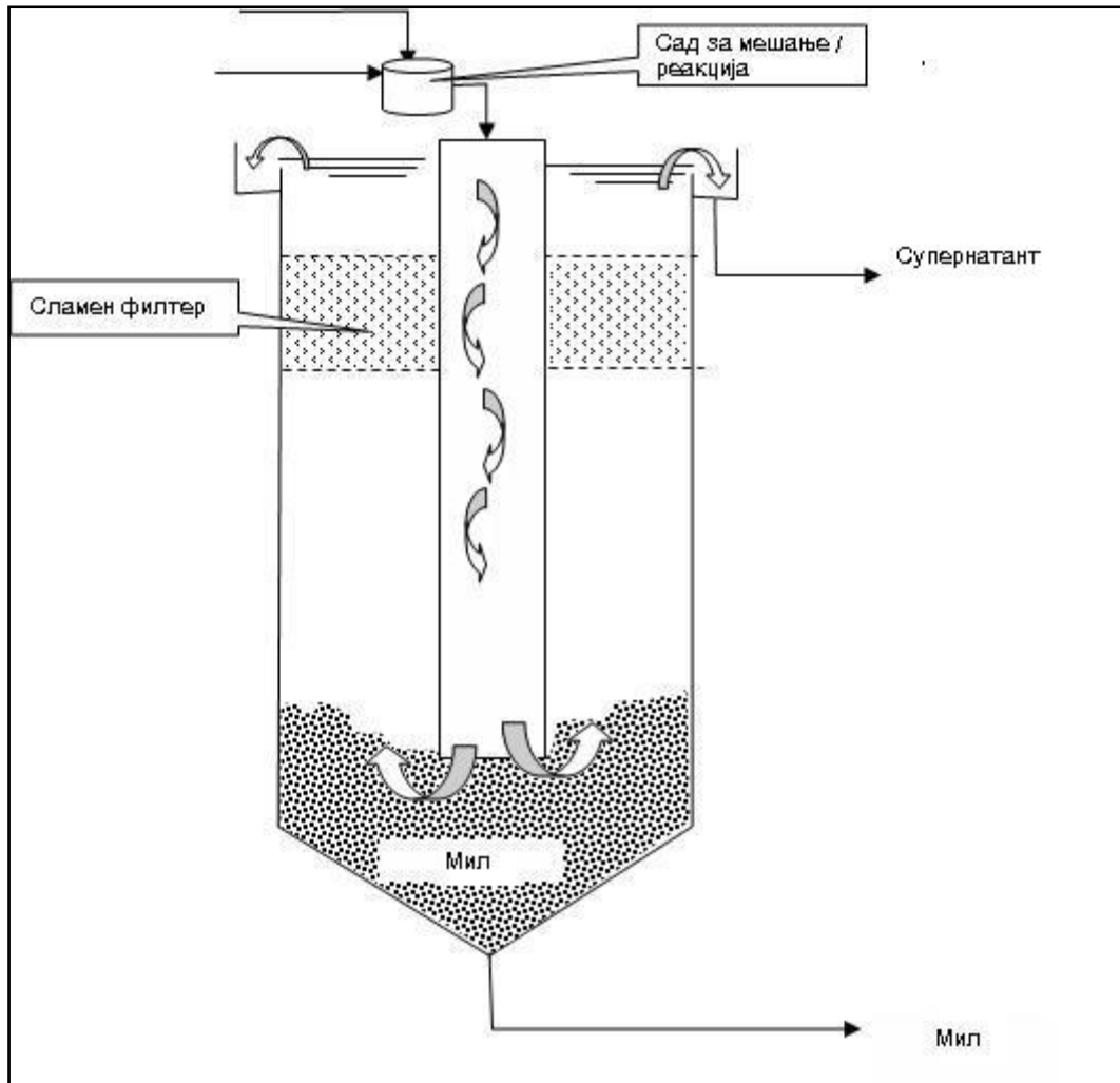
Слика 10 Преципитатор
