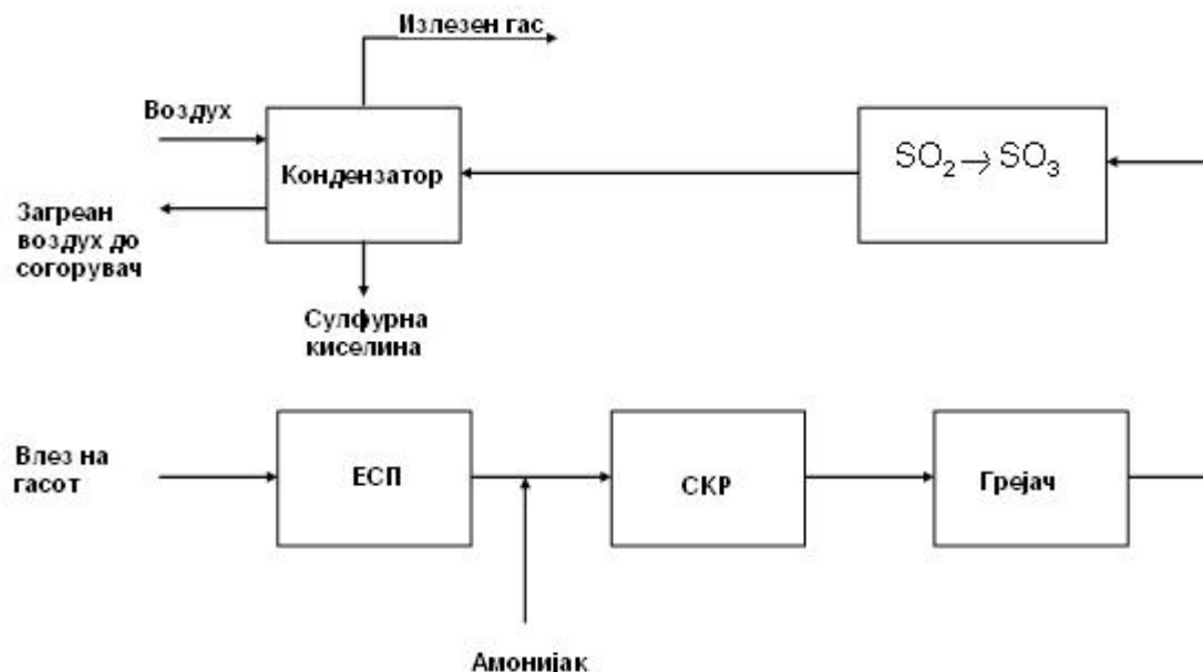
Слика 27 SNOx процес
