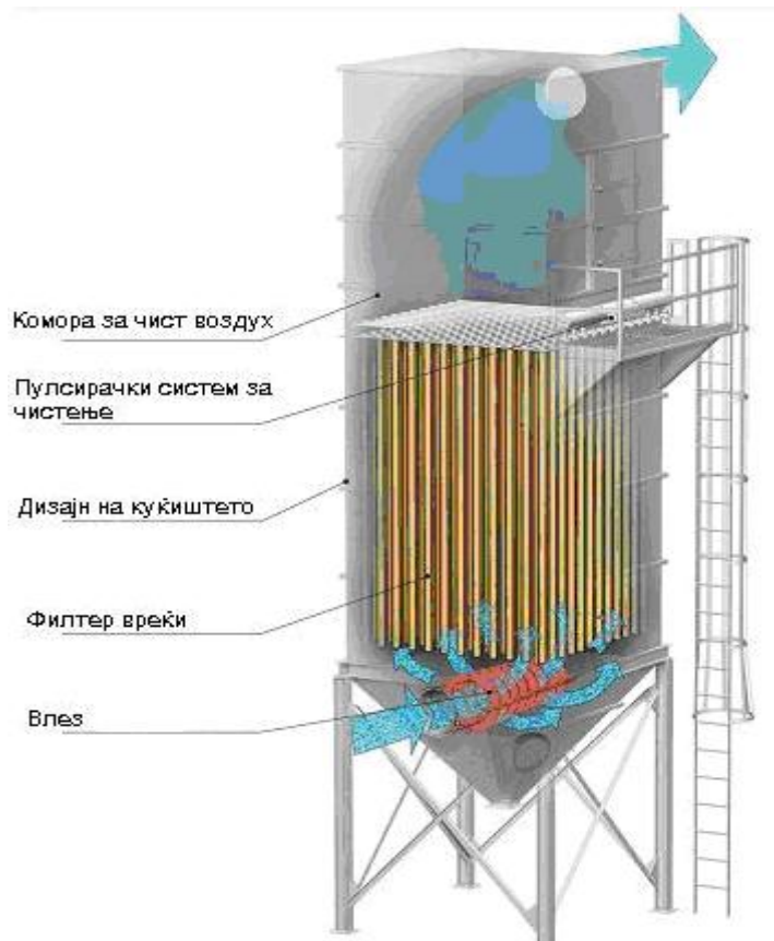
Слика 20 Составни делови на вреќаст филтер
